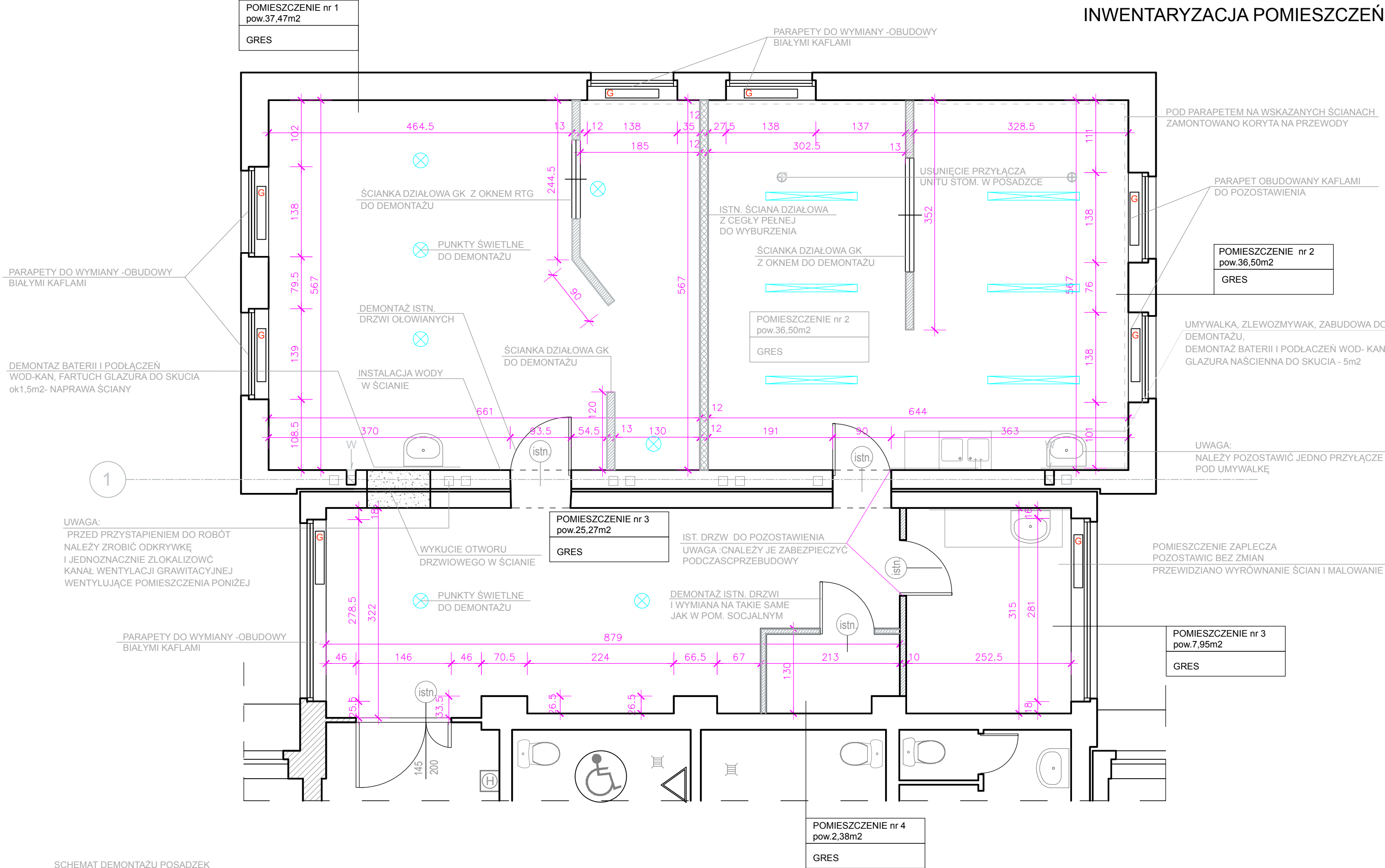
SCHEMAT DEMONTAŻU POSADZEK
